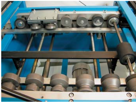
Цельные совместно обработанные каретки станка Dimos, модель Dipro-1S
