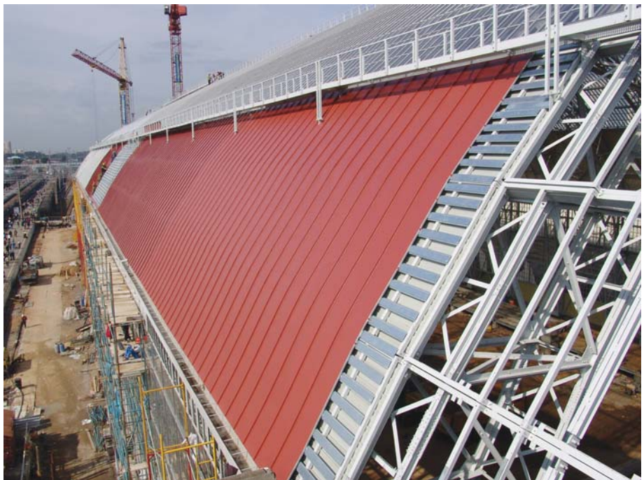
Фальцевая кровля с двойным стоячим фальцем (дебаркадер Киевского вокзала, г. Москва), выполненная на мобильном кровельном станке «МобиПроф», модель СФП-700
